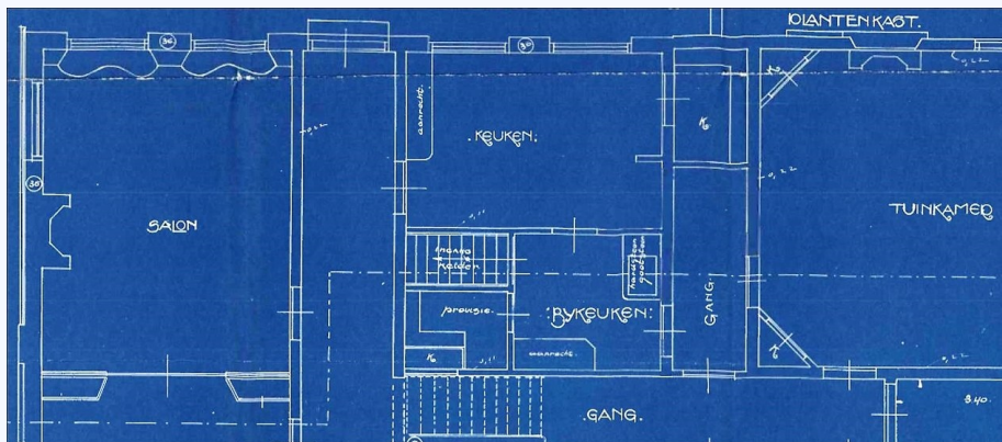
Plattegrond van de villa Blijdenstein begane grond met heel veel ruimte voor de keuken en bijkeuken.
