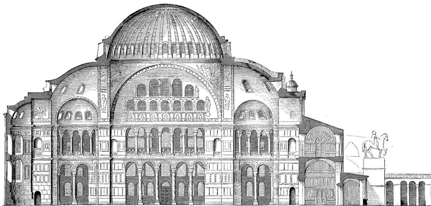
Doorsnee van de originele architectuur van de Hagia
