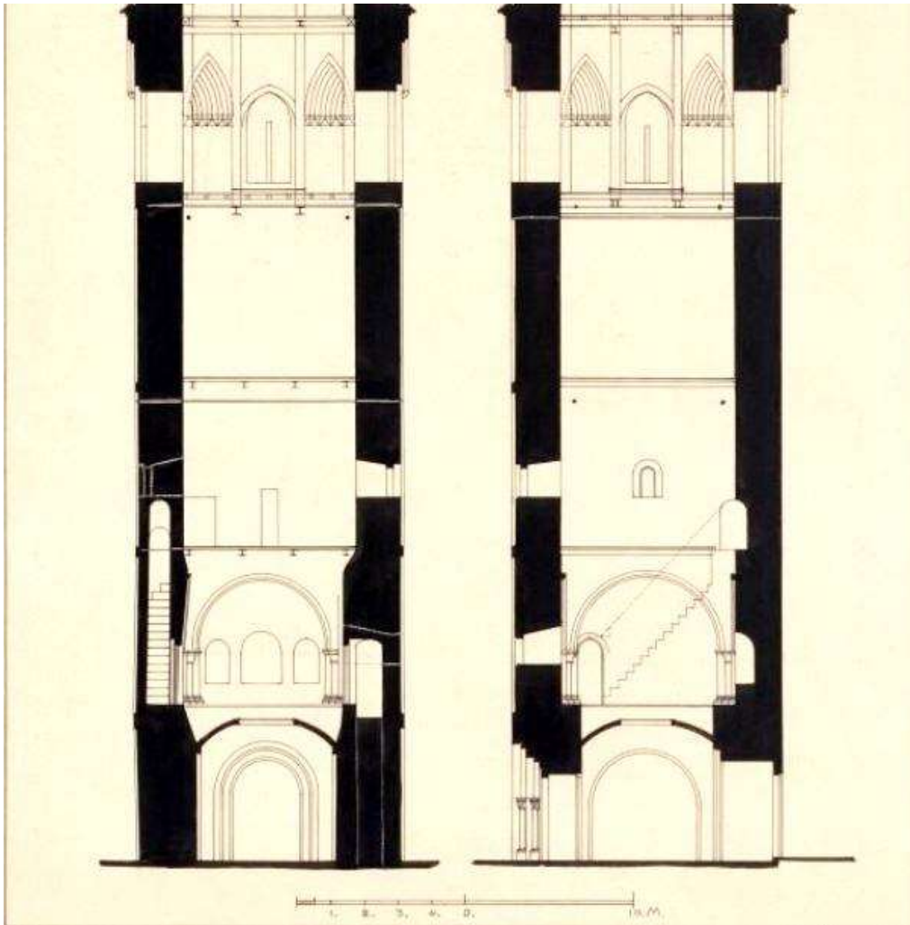
Doorsnede tekening van de toren uit 1925 van W. Scheepens waarin is weergegeven de inpandige trapstructuur naar de vermoedelijke St. Michaël kapel op de eerste etage.
